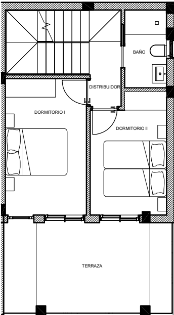
PLANTA -1 (NOCHE)
