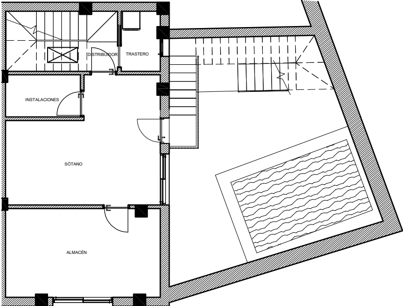
PLANTA SEMISÓTANO
